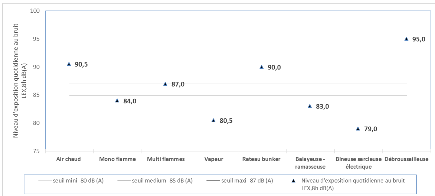
Figure 29 : Niveaux de bruit en fonction du matériel - comparaison aux valeurs réglementaires
