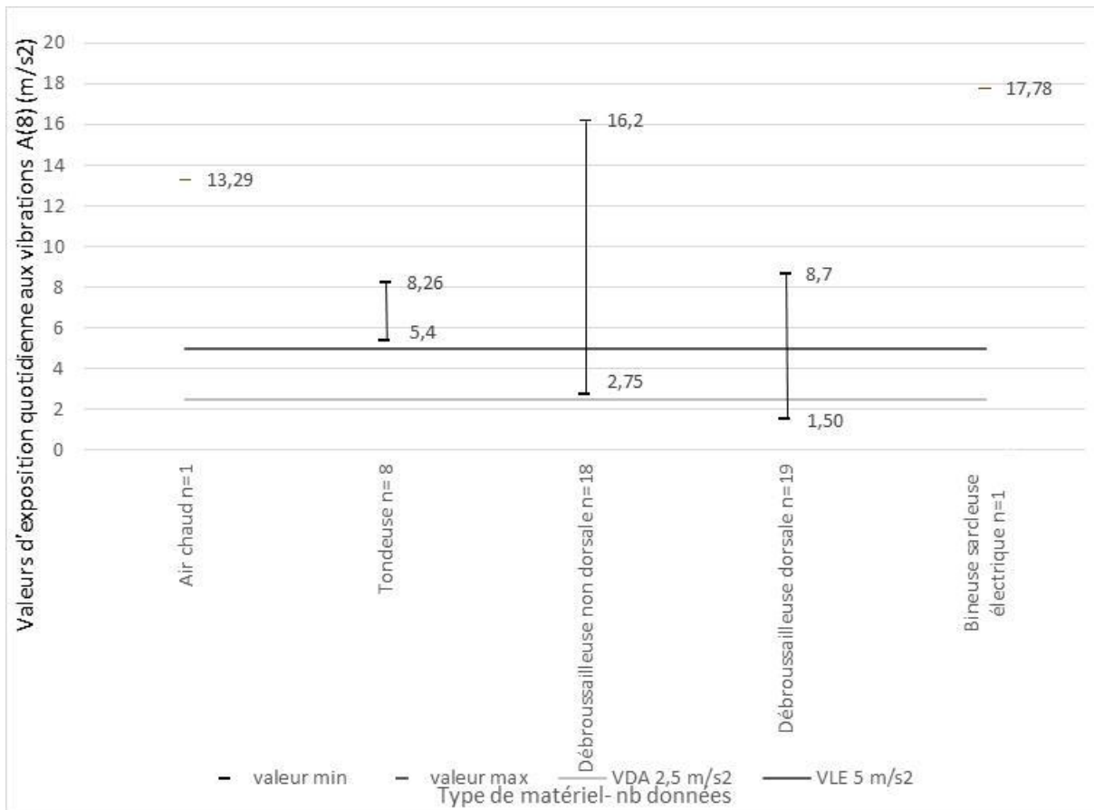
Figure 13 : Niveaux d'exposition aux vibrations main bras en fonction du matériel - comparaison aux valeurs réglementaires
