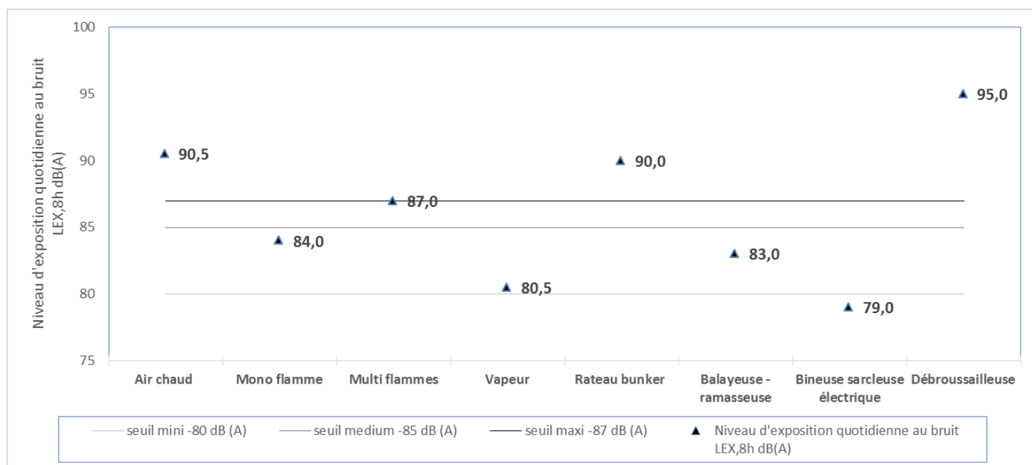
Figure 10 : Niveaux de bruit en fonction du matériel - comparaison aux valeurs réglementaires
