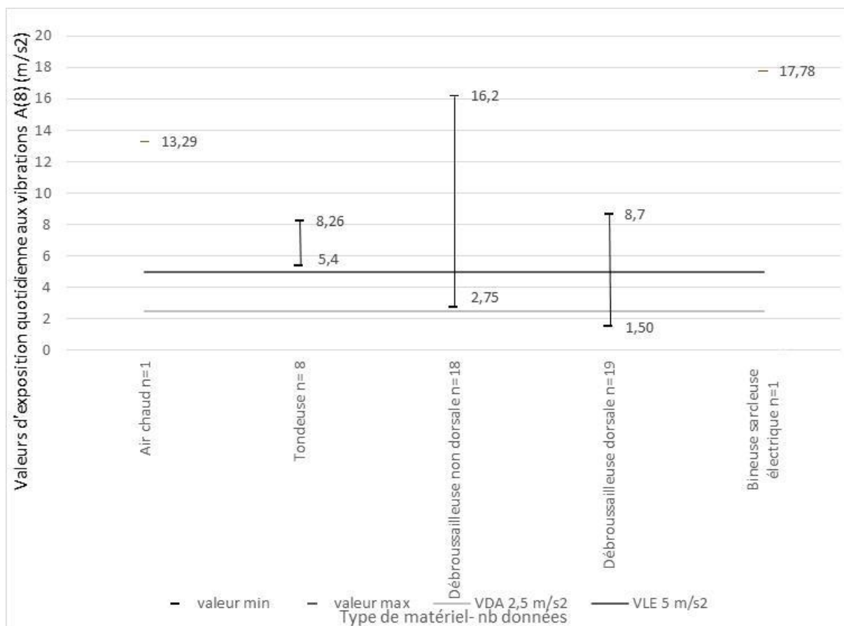
Figure 32 : Niveaux d'exposition aux vibrations main bras en fonction du matériel - comparaison aux valeurs réglementaires
