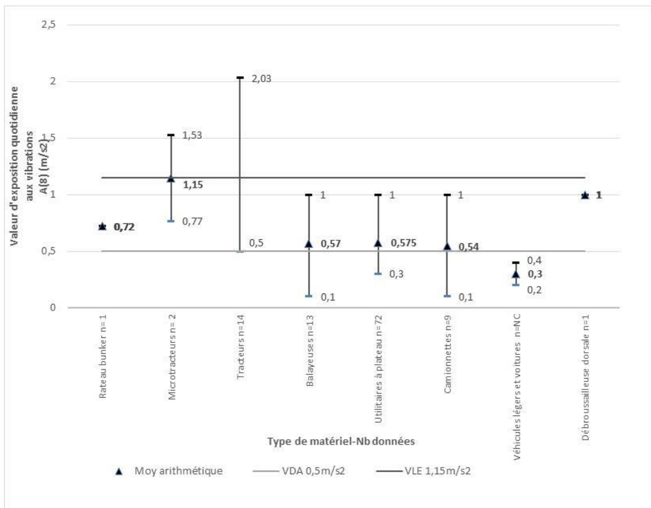
Figure 30 : Niveaux d'exposition aux vibrations corps entier en fonction du véhicule ou du matériel - comparaison aux valeurs réglementaires
