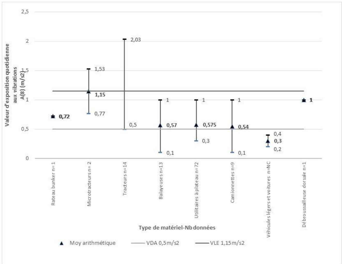
Figure 11 : Niveaux d'exposition aux vibrations corps entier en fonction du véhicule ou du matériel - comparaison aux valeurs réglementaires
