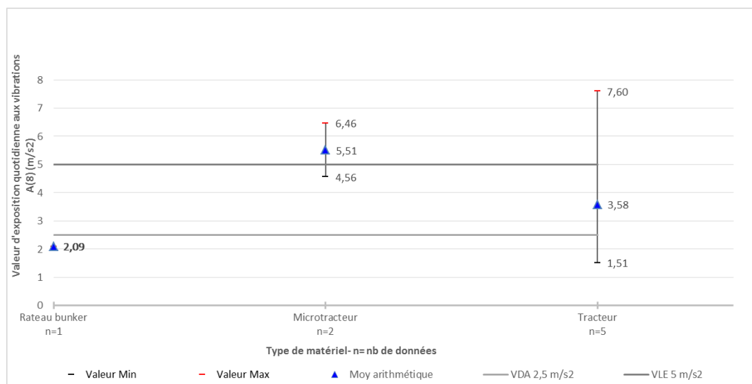
Figure 31 : Niveaux d'exposition aux vibrations main bras en fonction du véhicule - comparaison aux valeurs réglementaires
