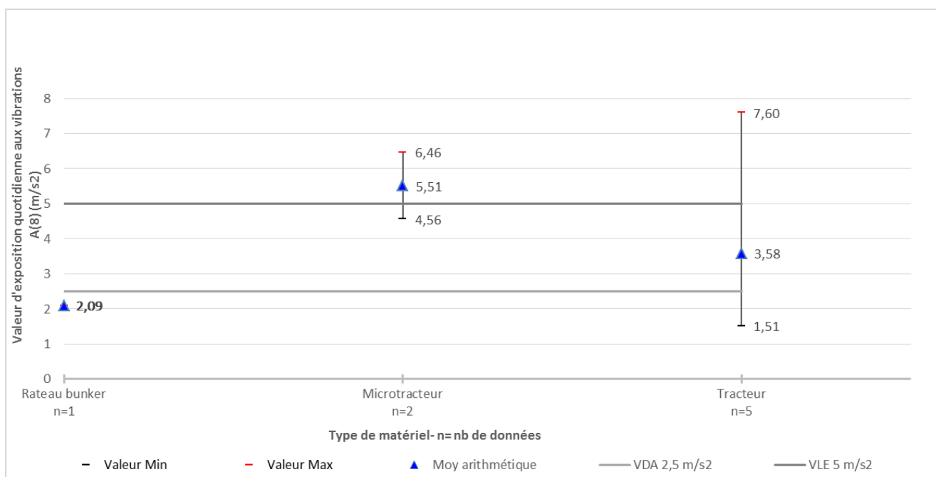
Figure 12 : Niveaux d'exposition aux vibrations main bras en fonction du véhicule - comparaison aux valeurs réglementaires
